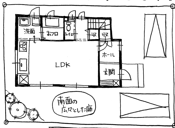
配置図兼1F平面図
